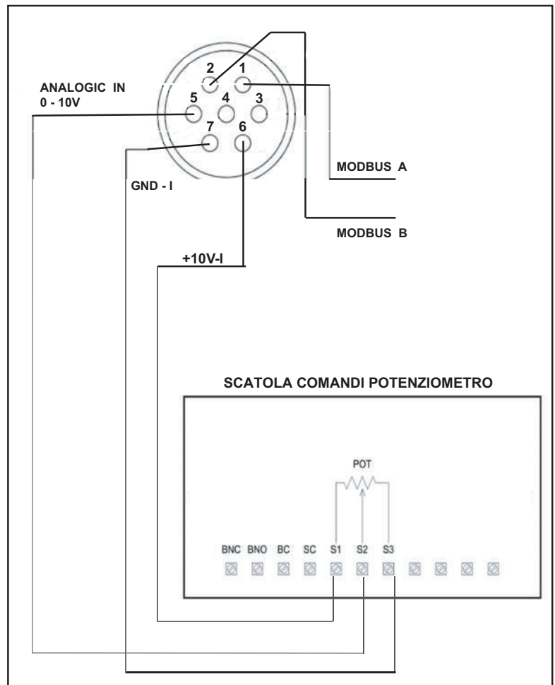
DETTAGLIO CONNESSIONI
